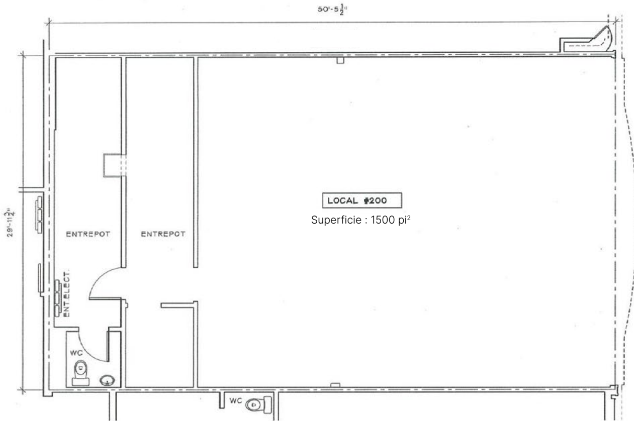
VUE EN PLAN DU LOCAL NO:200 3/16"=1'-0"
