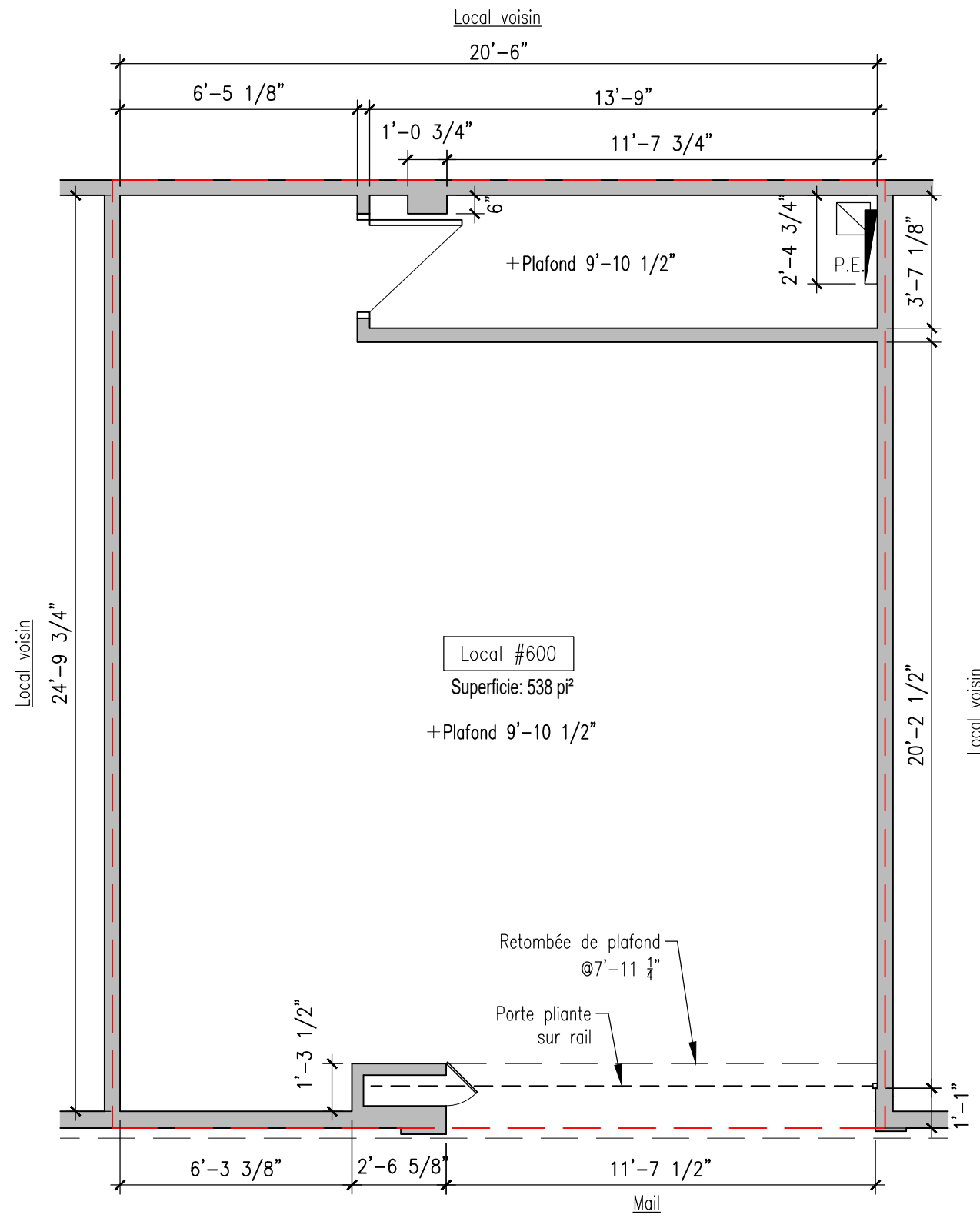
Local #600 ÉCHELLE 1/4" = 1'-0"
