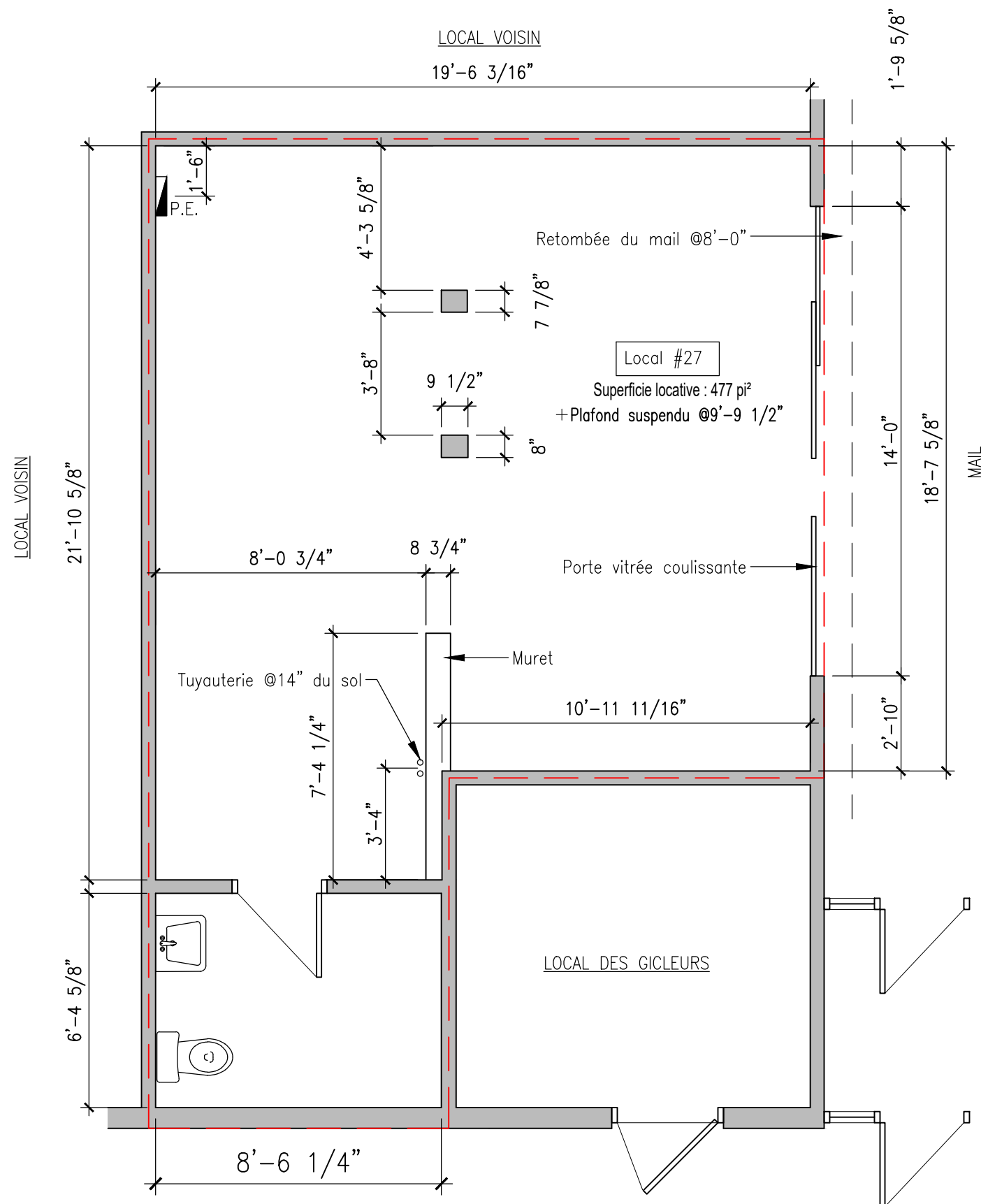
Local #27 ÉCHELLE 1/4" = 1'-0"
